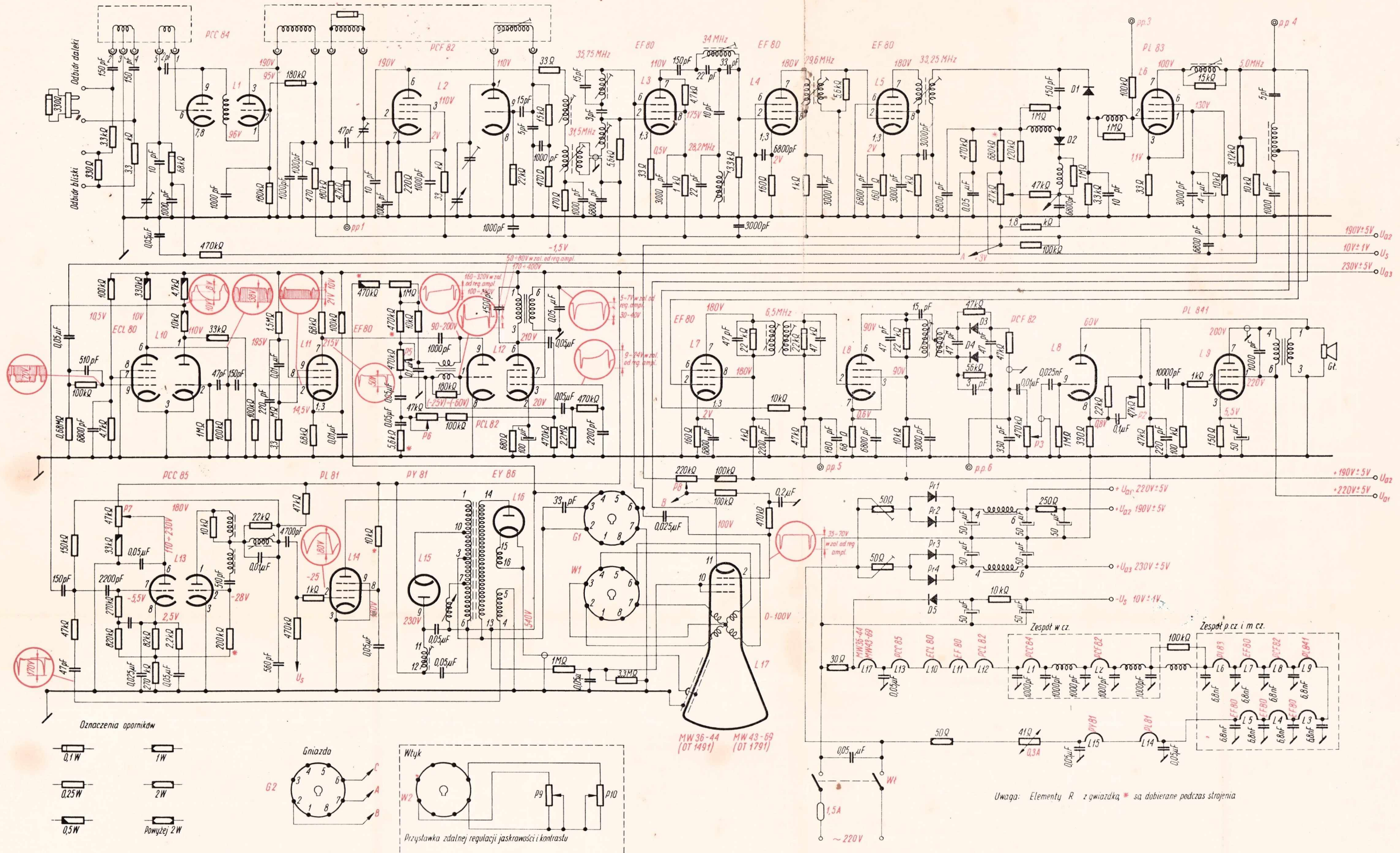
Schemat 1. Odbiornik telewizyjny Turkus (Jantar i Szmaragd)
