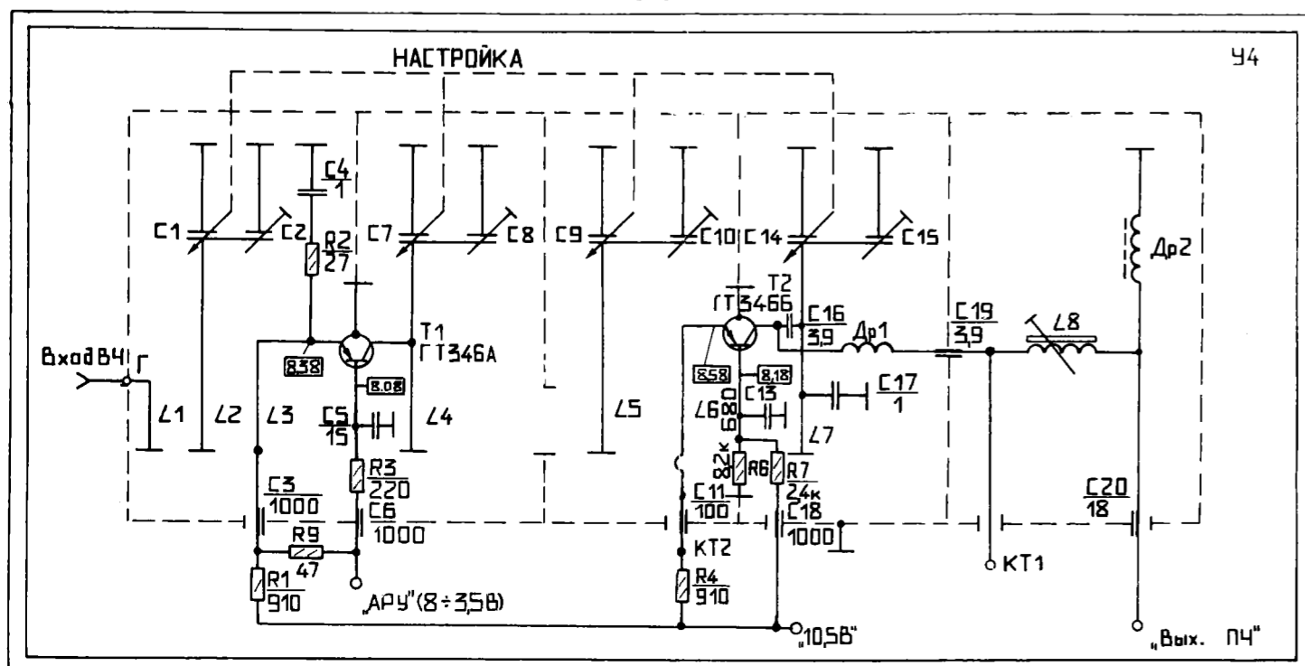
Схема селектора телевизионных каналов дециметровых волн— СК—Д—20
