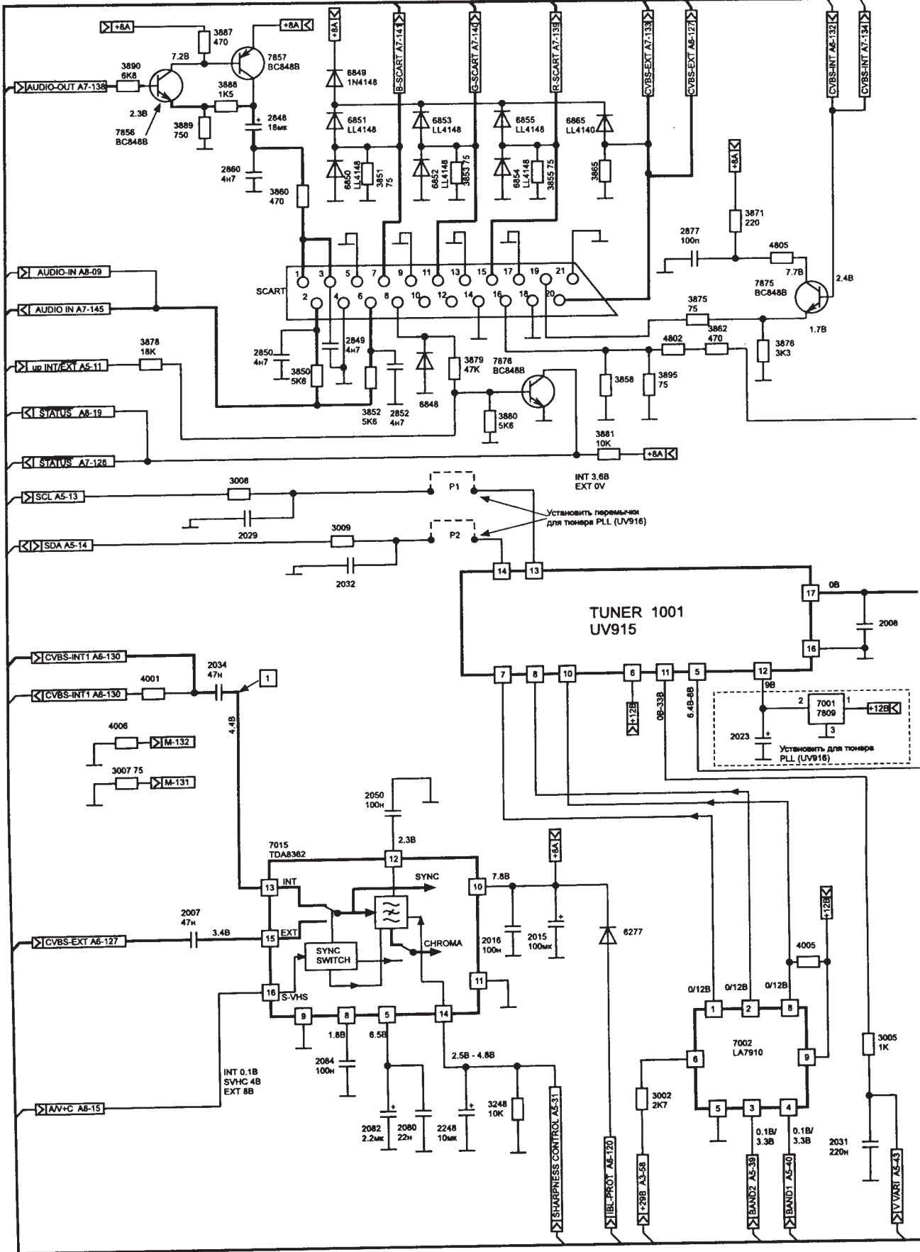
Принципиальная схема. Радиоканал
