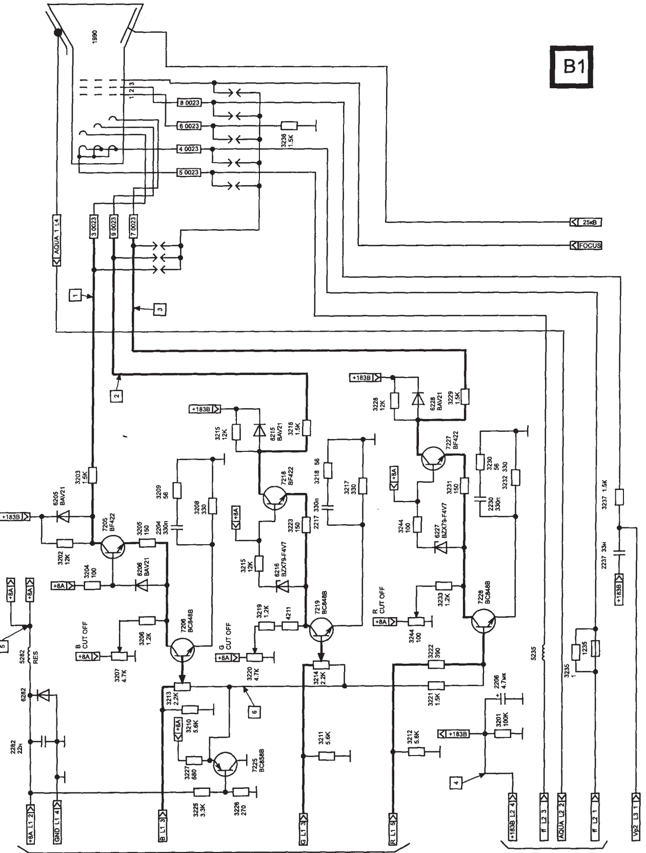
Принципиальная схема. Плата кинескопа
