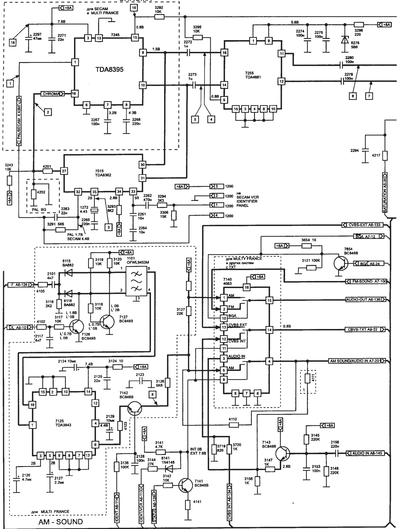
Принципиальная схема. Декодер PAL/SECAM. Переключатель AV/TV
