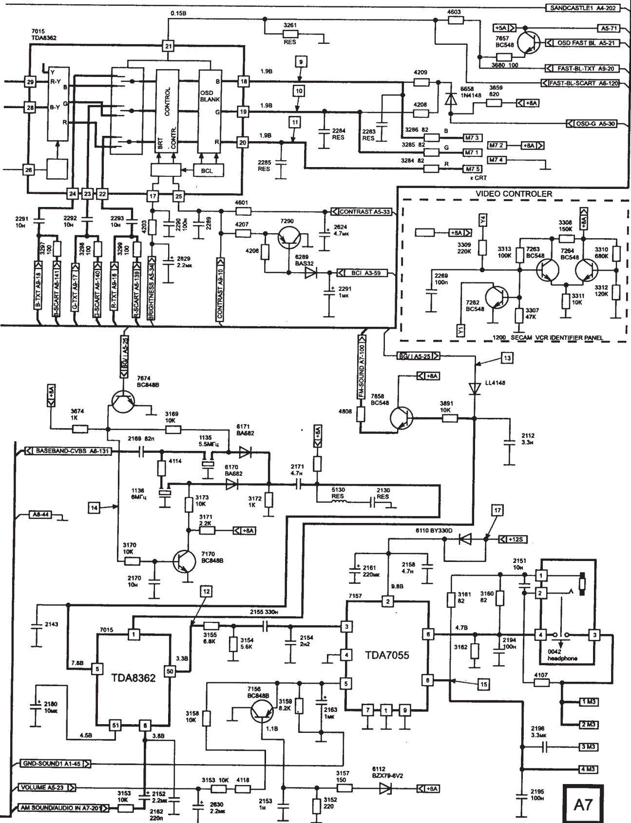
Принципиальная схема. Видеопроцессор. Усилитель звуковой частоты
