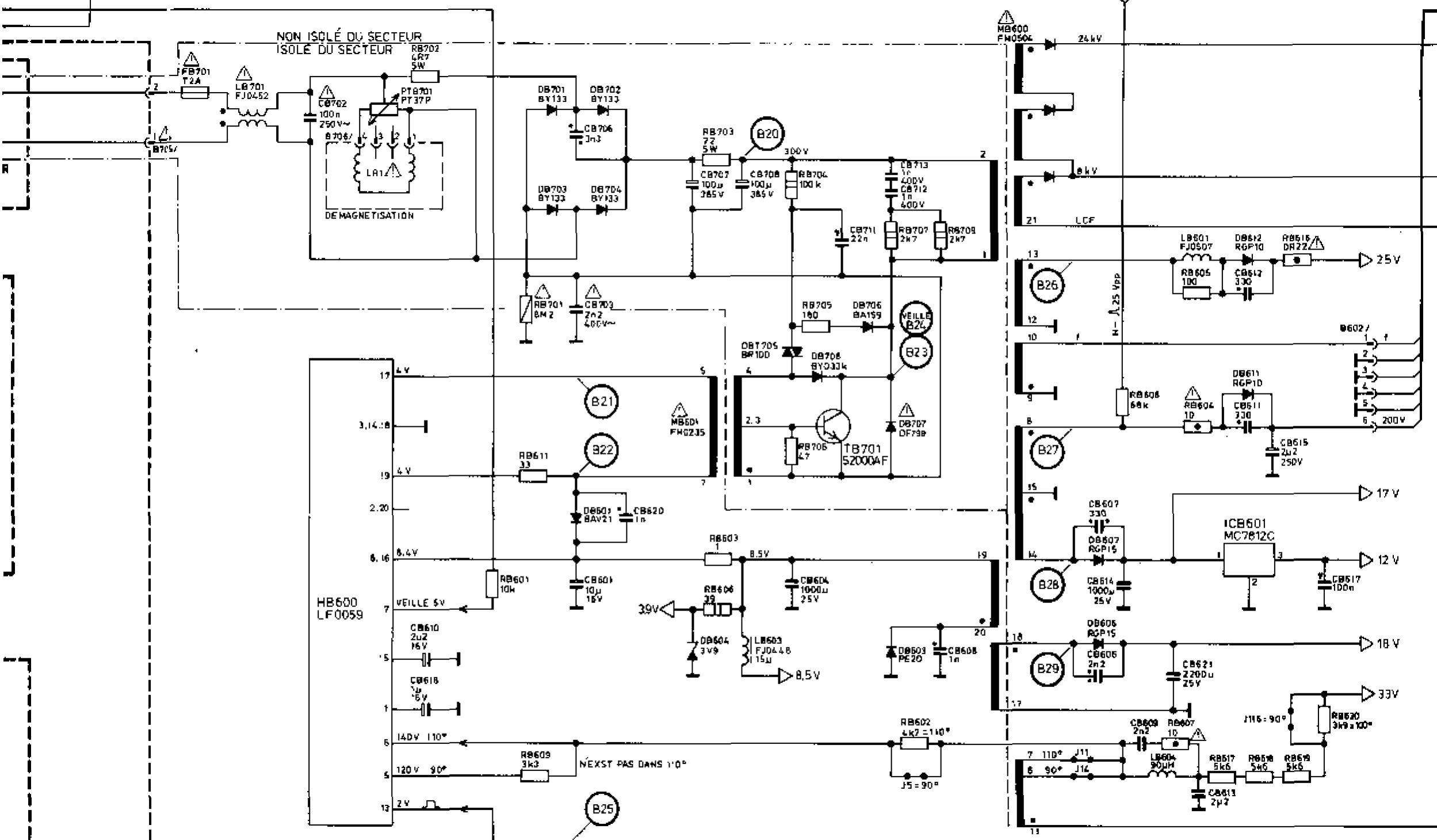
STB 189 C (90°) PLATINE DE BASE
