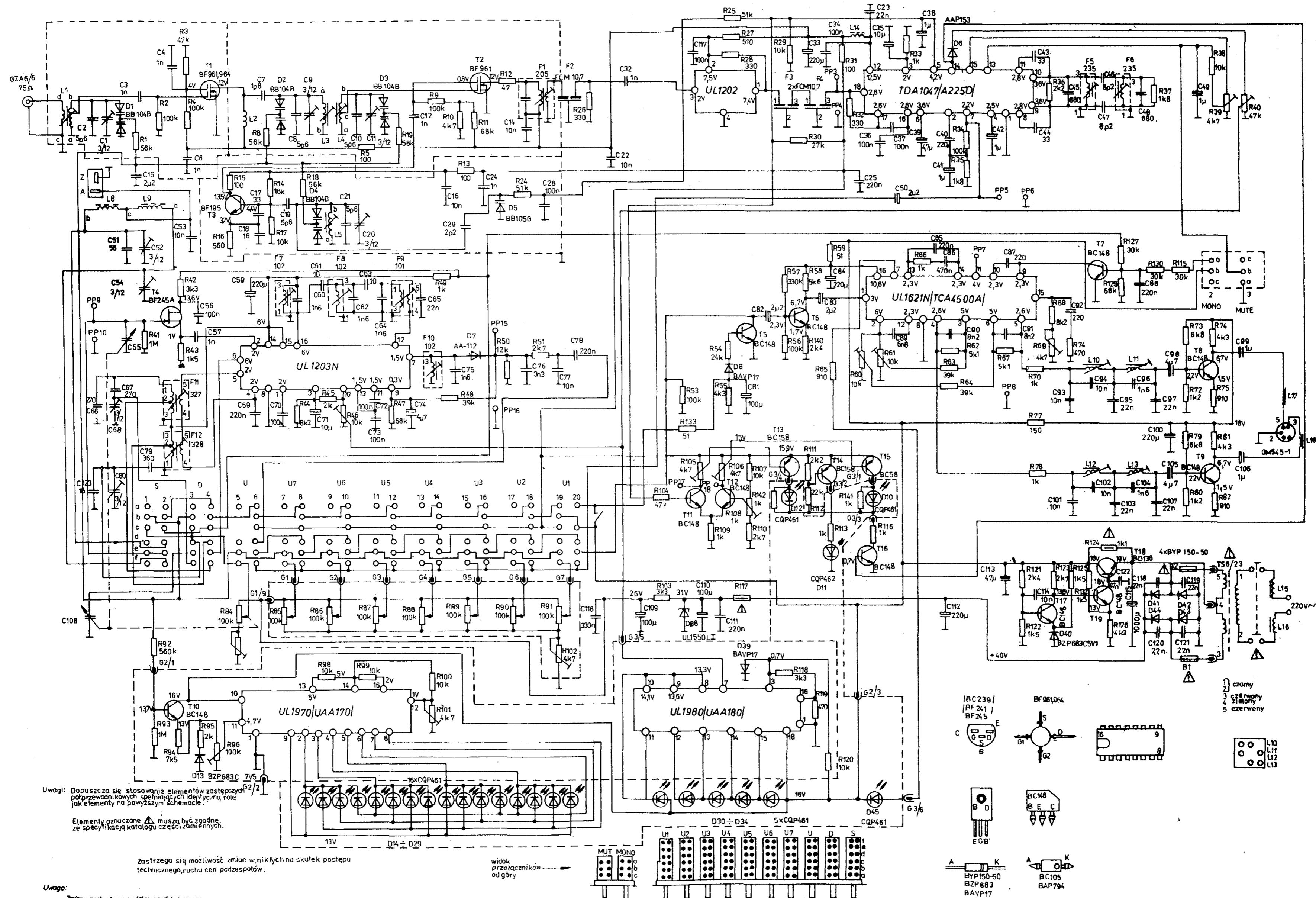
Schemat ideowy tunera T-9015
