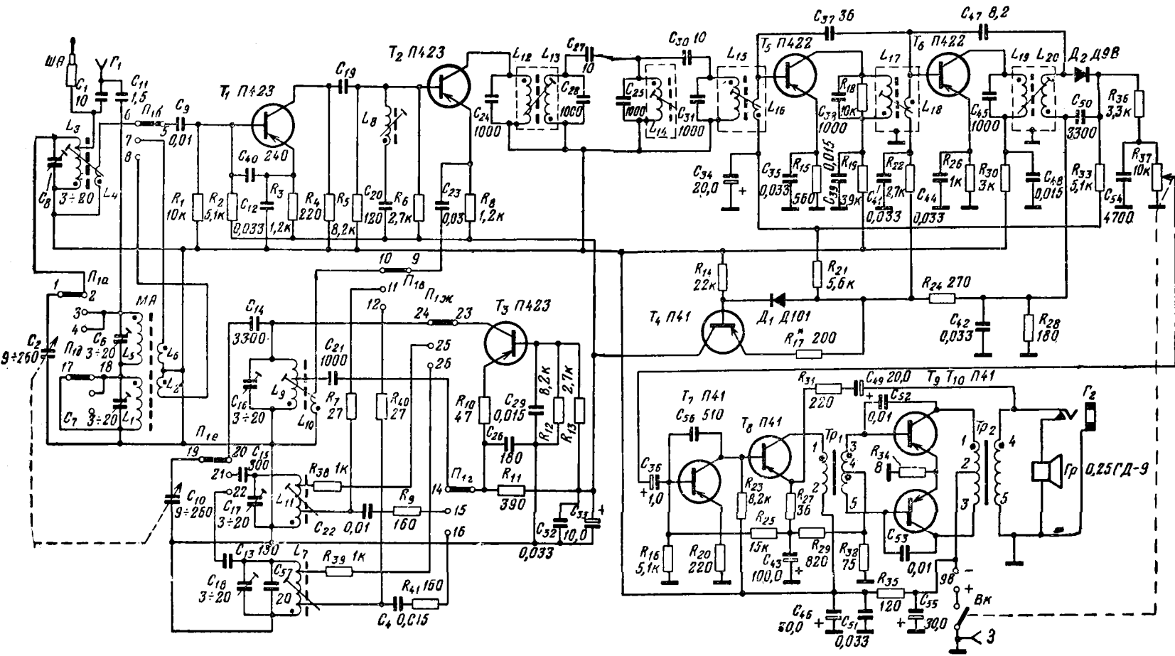
Принципиальная схема приемника «Банга». Переключатель диапазонов установлен в положение КВ.
