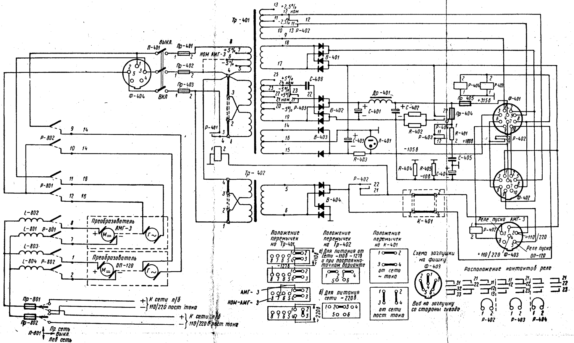
Принципиальная схема выпрямительного блока радиостанции „Акация“
