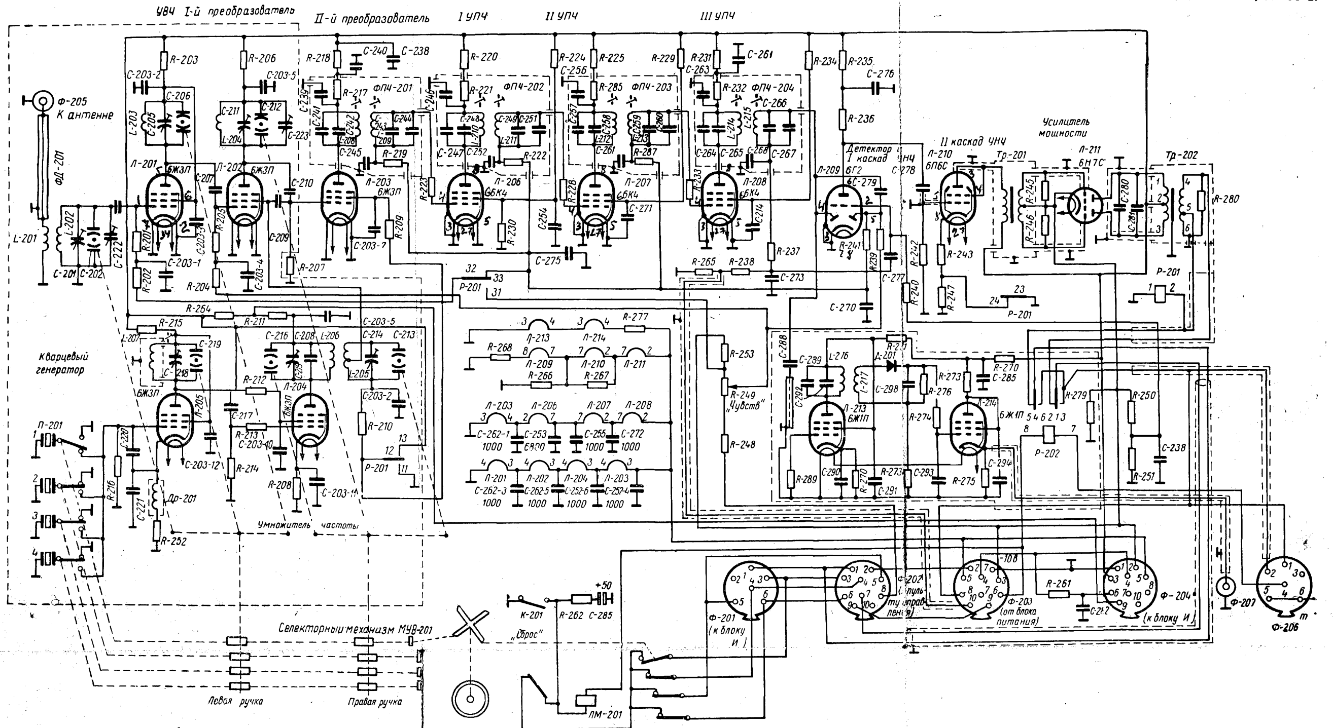
Принципиальная схема приемника радиостанции „Акация“
