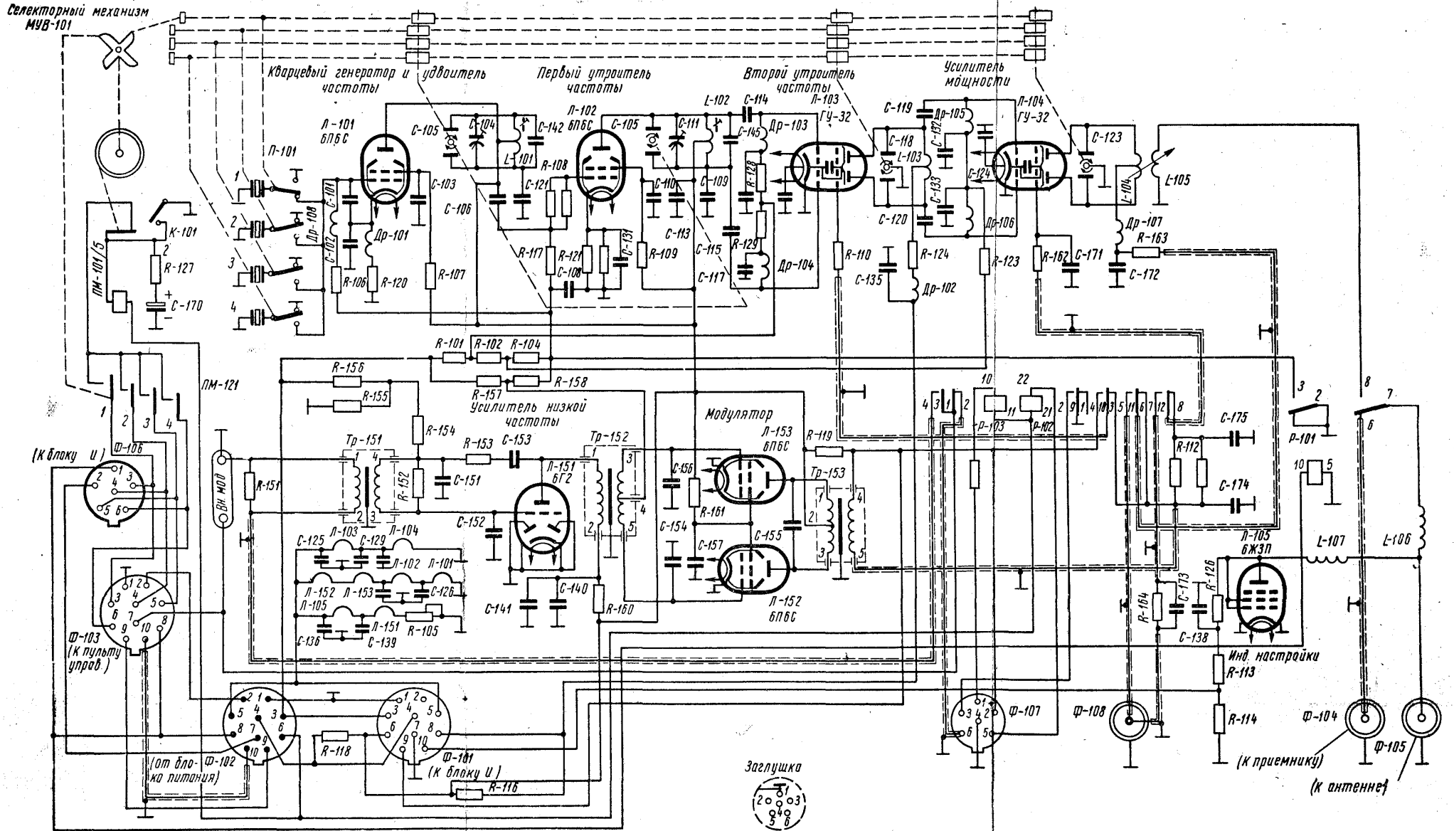
Принципиальная схема передатчика радиостанции „Акация“
