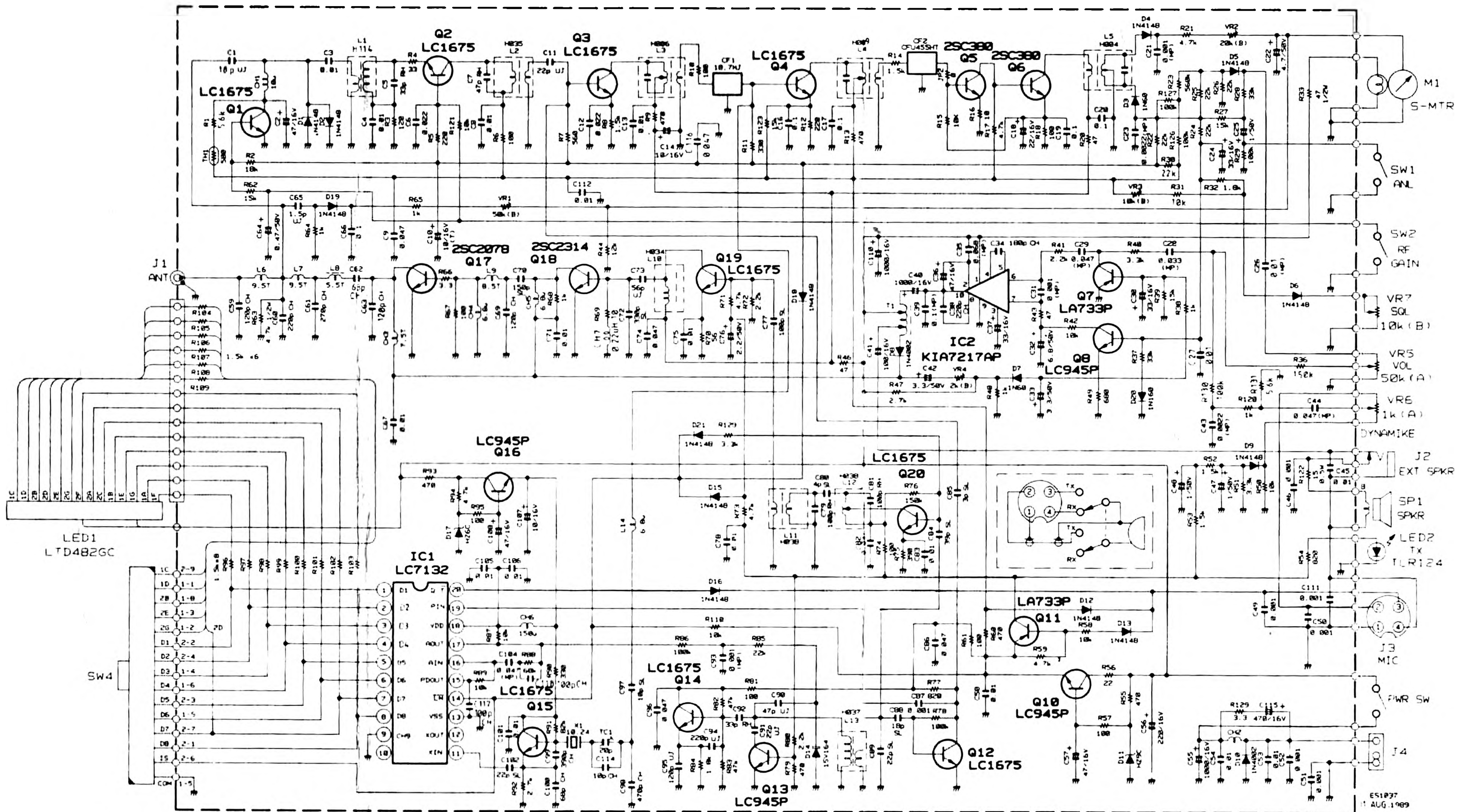
Schemat ideowy radiotelefonu Cobra 21 LTD Classic
