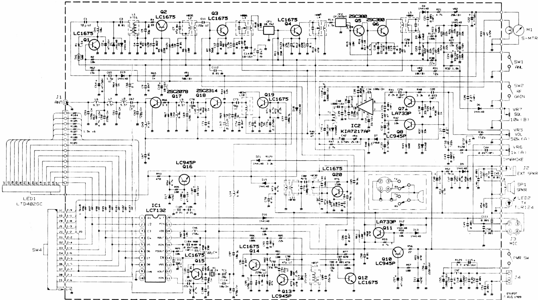
Rys. 11.15. Schemat ideowy radiotelefonu Cobra 21 LTD Classic
