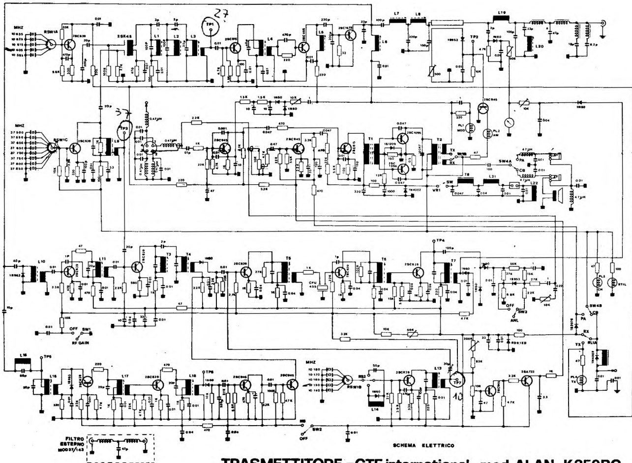
TRANSMETTITORE -CTE international-mod. ALAN K350BC
