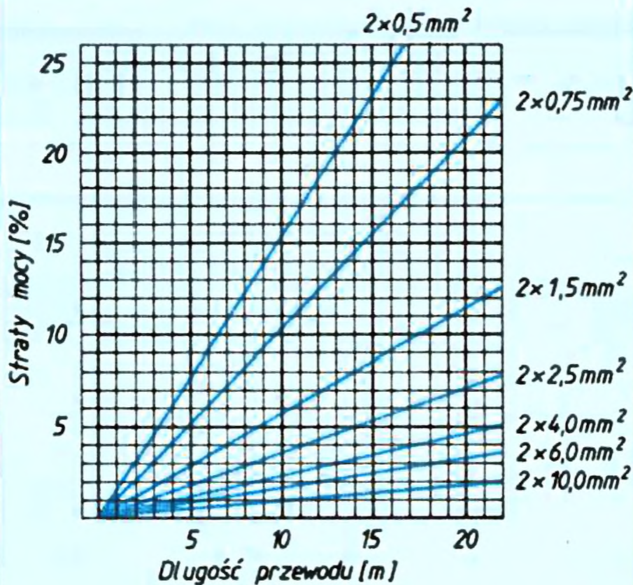
Wykres straty mocy w funkcji długości przewodu głośnikowego dla różnych powierzchni przekrojów przewodu
