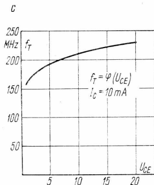
Rys. 2. Charakterystyki tranzystorów grupy BF504-506
