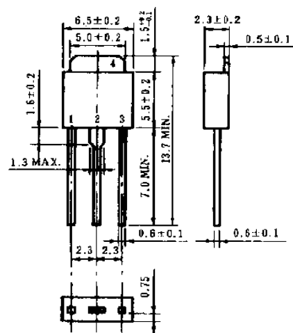
MP-3
