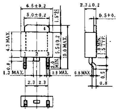
MP-3Z
