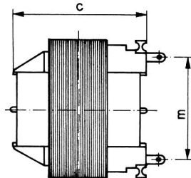
Transformator poz. 1÷5 i 7,8
