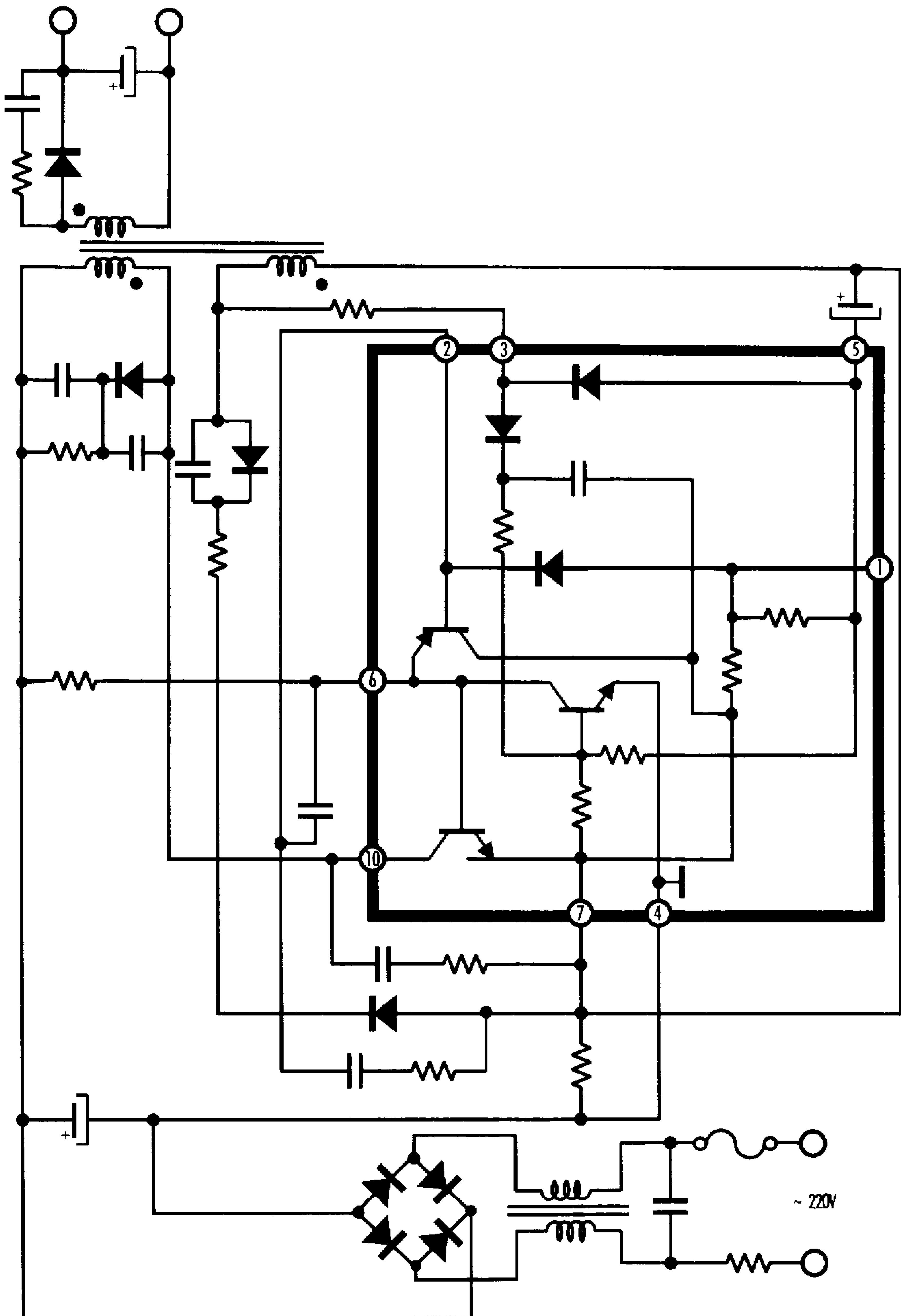
Rys. 76. Aplikacja układu STK 73600
