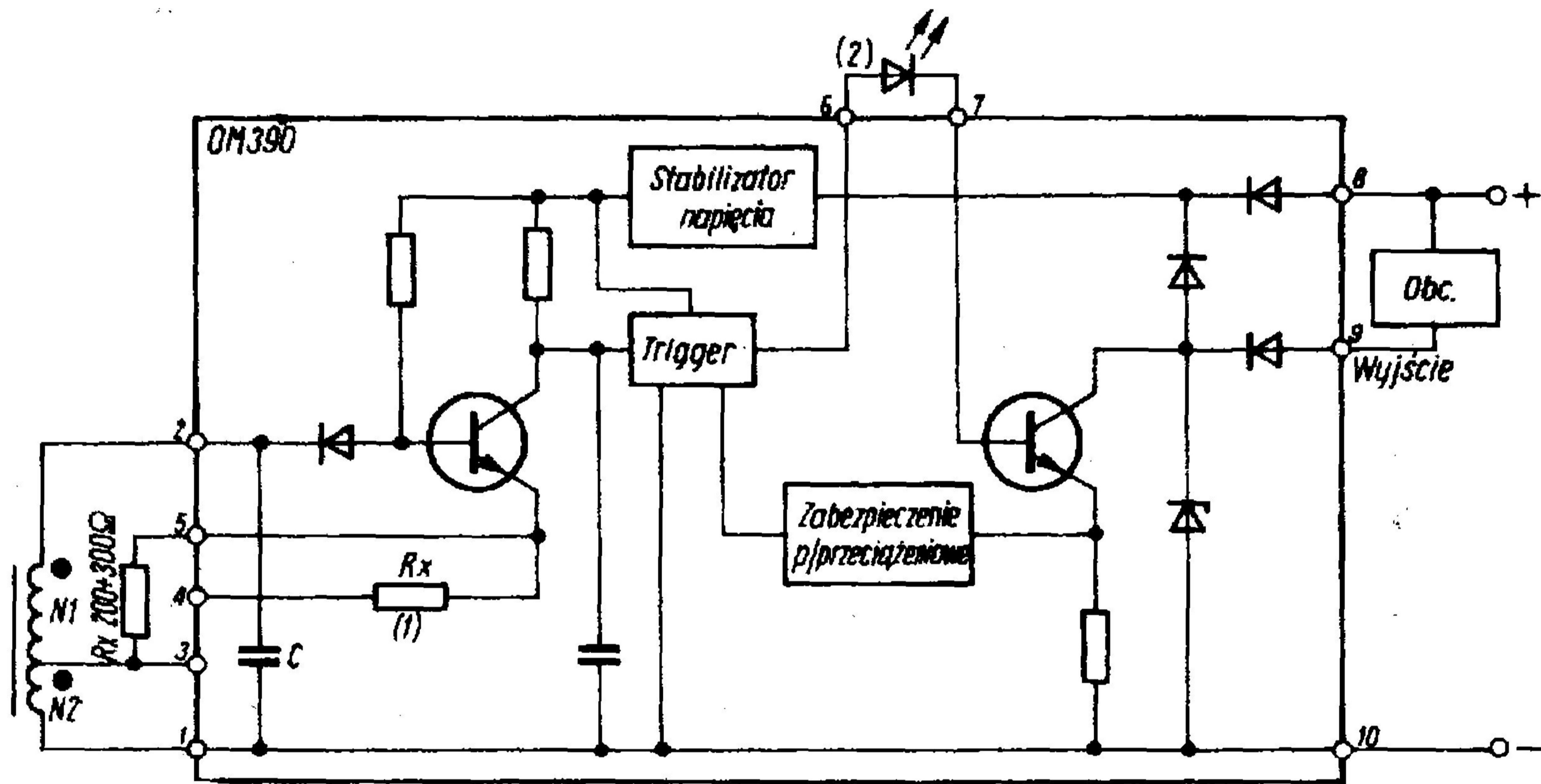
Schemat hybrydowego układu scalonego OM390 (Philips)
