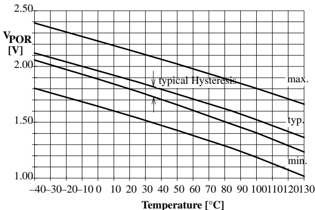
Figure 8. Temperature versus V POR
