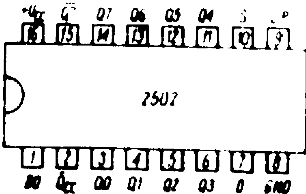
Рис. 8. Микросхема выводов режима асинхронного переключения
