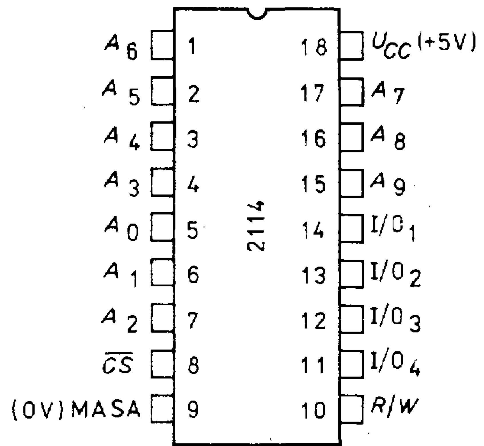
Rys. 7.14. Moduł pamięci RAM 2114: a) rozkład wyprowadzeń; b) symbol logiczny
