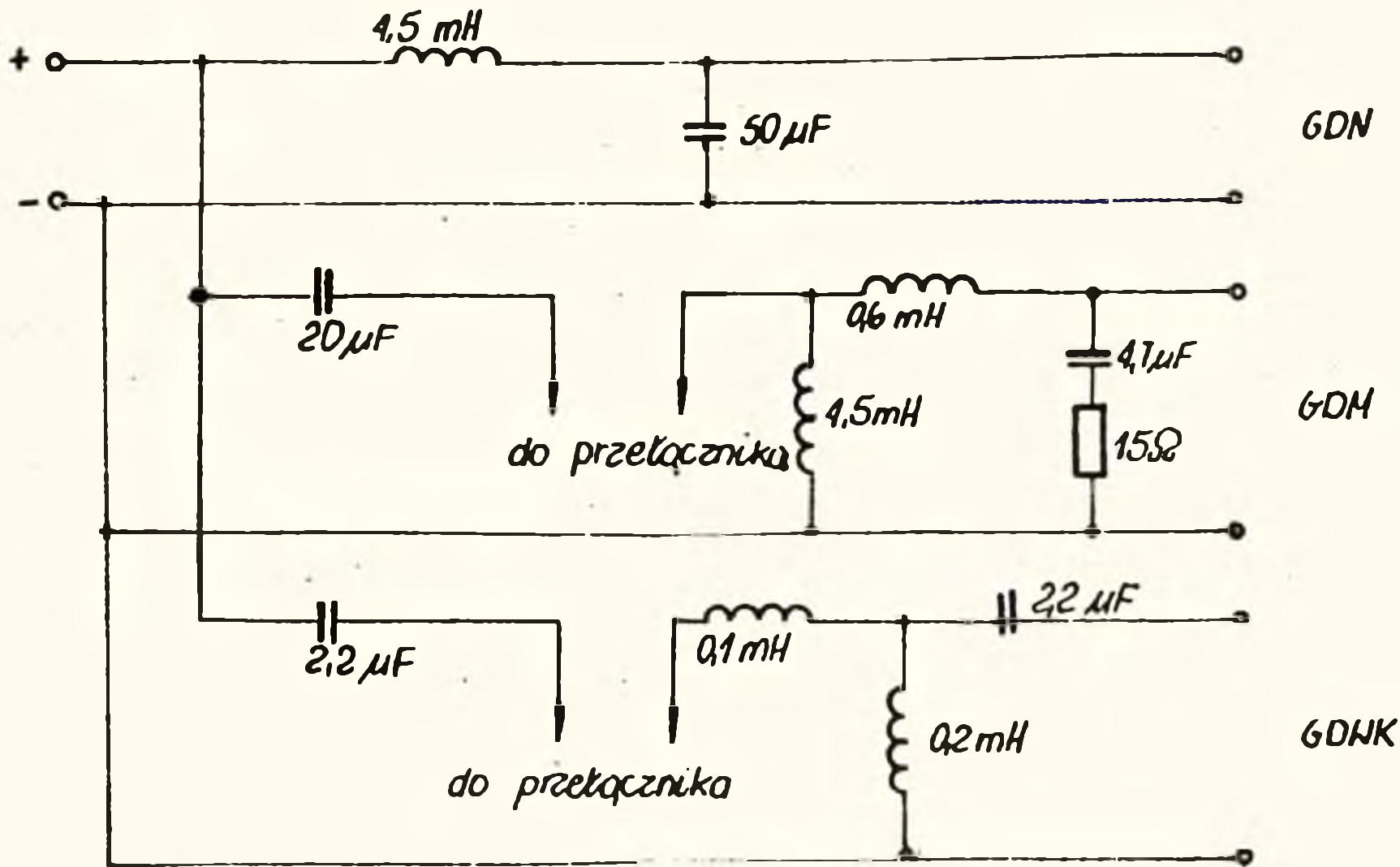
Schemat elektryczny przetwornicy ZGBOC115.
