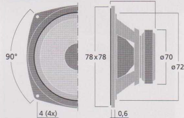
SPH-75/8
