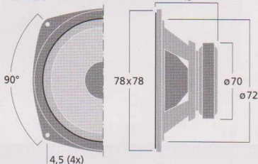
SP-45/8
