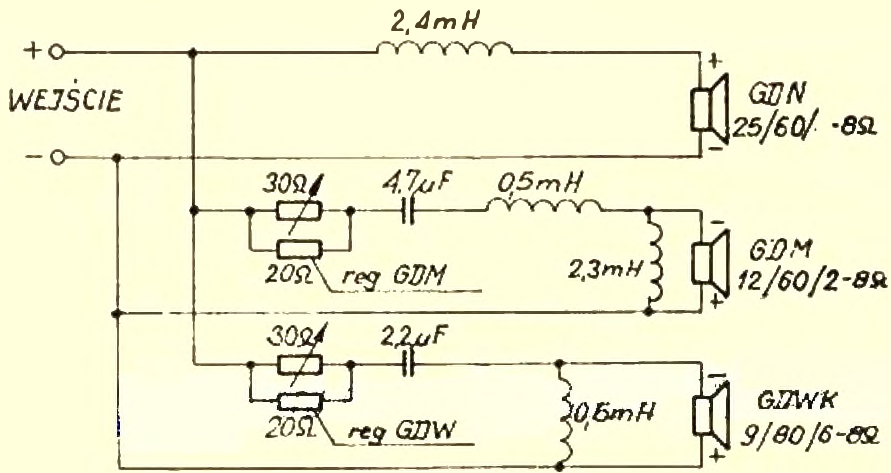
Schemat ideowy zestawu ZgB 80-8-693
