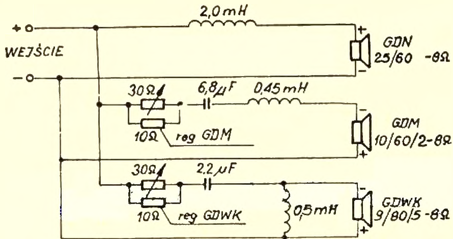
Schemat ideowy zestawu ZgB-70-8-693
